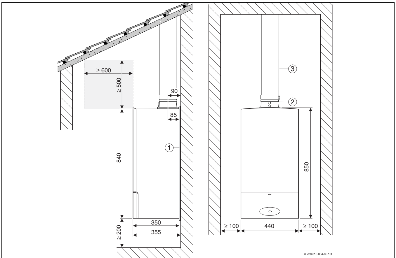
sl. 8 Ø 80/125 mm, kosi krov
