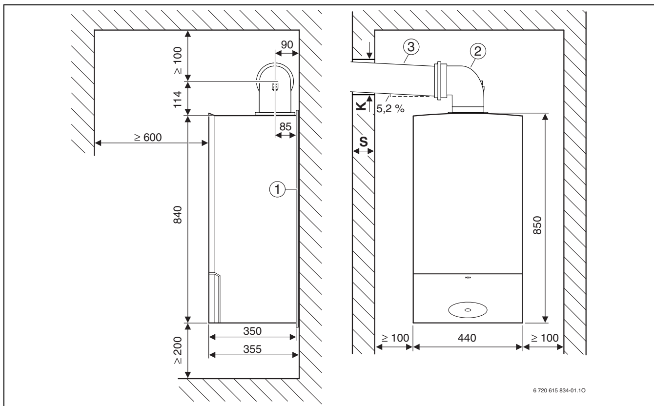
sl. 5 Dimovod \varnothing 80/125 mm ili \varnothing 80 mm
