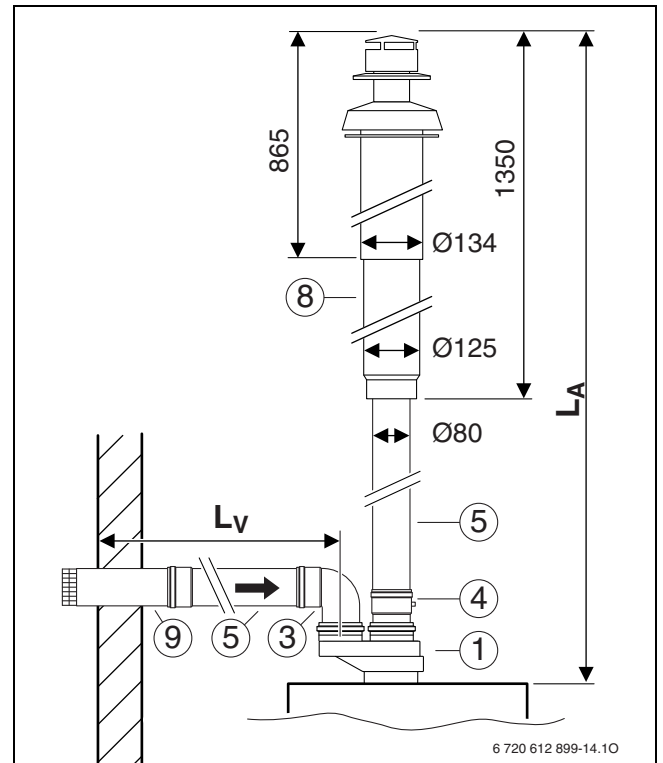
sl. 16 Vođenje izduvnih gasova po C 52
